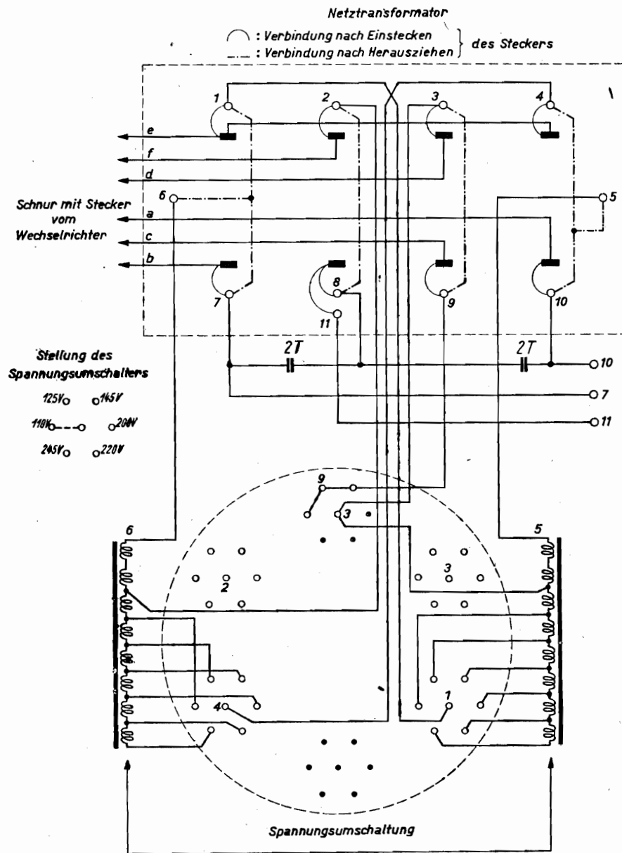
Philips Wechselrichter Typ 7926
