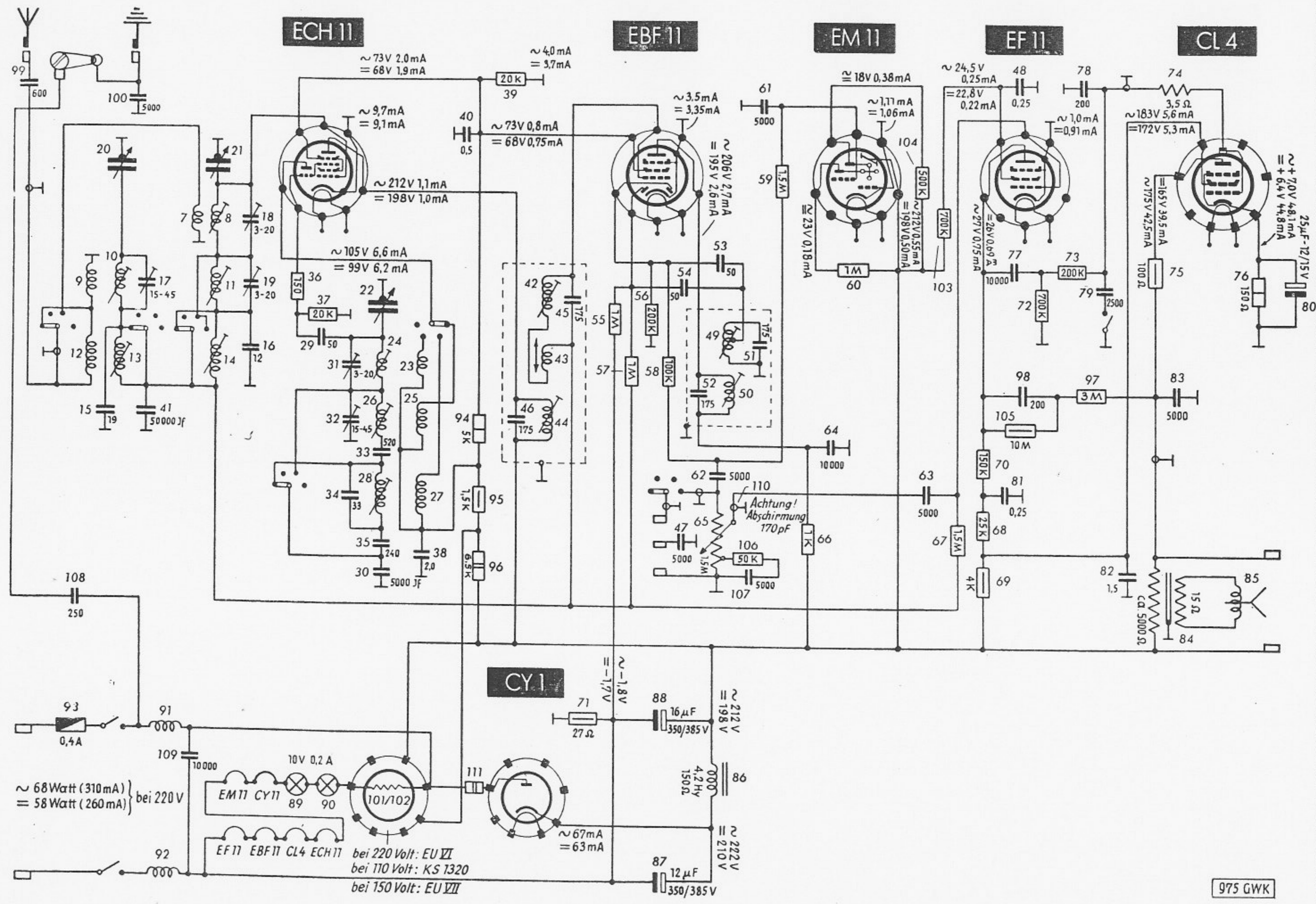
Schalbild
